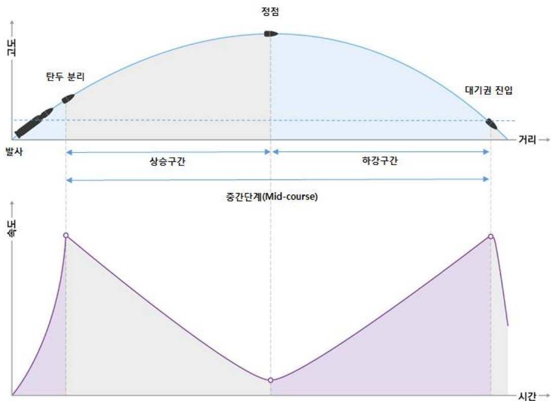
[그림 4] 미사일 발사 후 발사의 고도와 구간별 속도 변화 개념도
