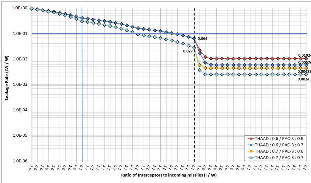
[그림 23] 사드: 3 발, PAC-3: 2 발 (SSPk: 0.6~0.7, W=100)
