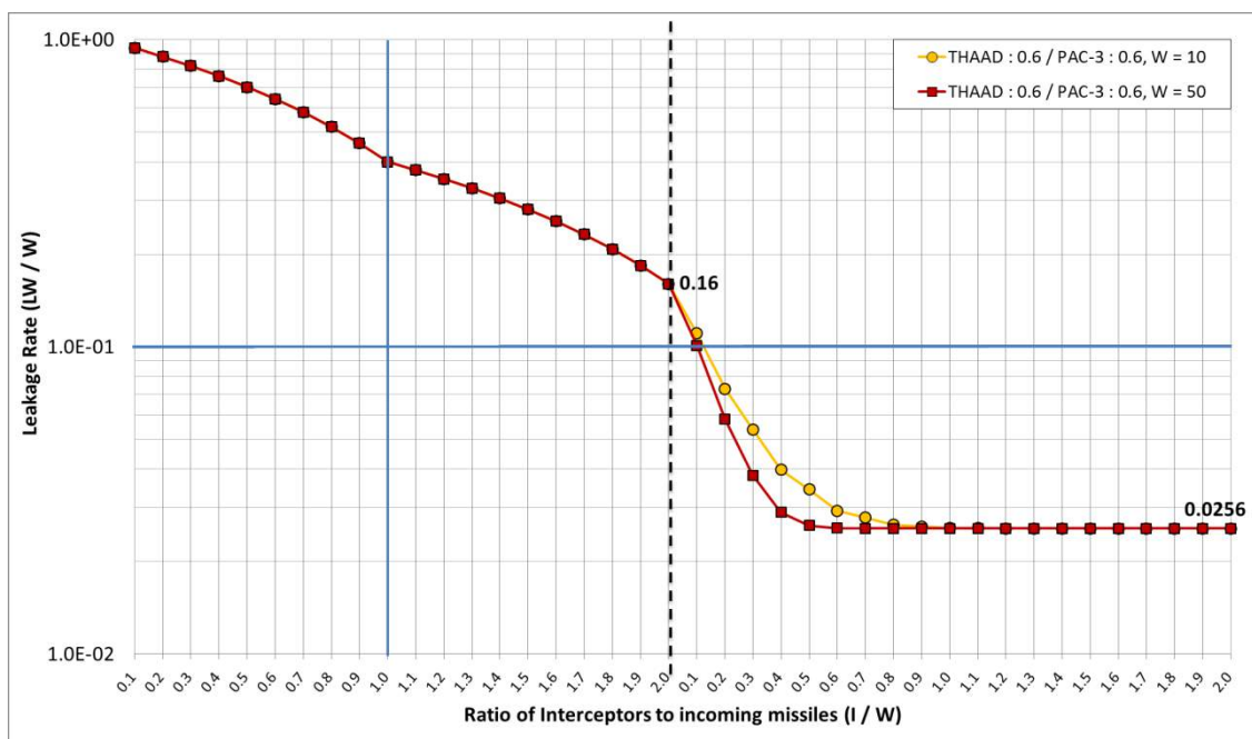
[그림 17] 적 미사일 수가 다를 경우 leakage rate 그래프 모양 변화 ( W=10, 50 )
