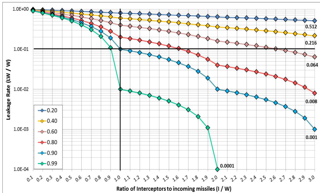
[그림 11] Tier-1 에서 다양한 SSPk 에 대한 leakage rate 그래프
