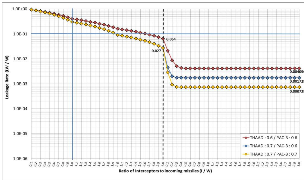
[그림 24] 사드: 3 발, PAC-3: 3 발 (SSPk: 0.6~0.7, W=100)
