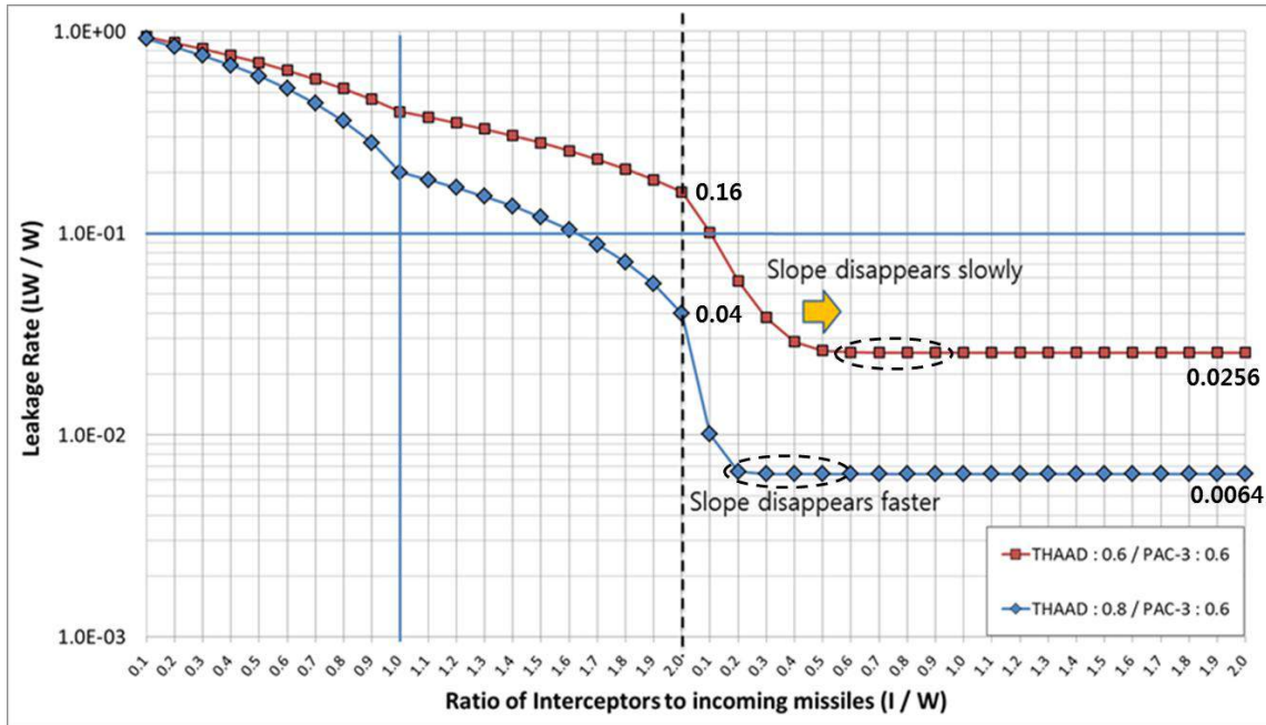
[그림 14] 사드의 SSPk가 다를 경우 leakage rate 그래프 (W=50)
