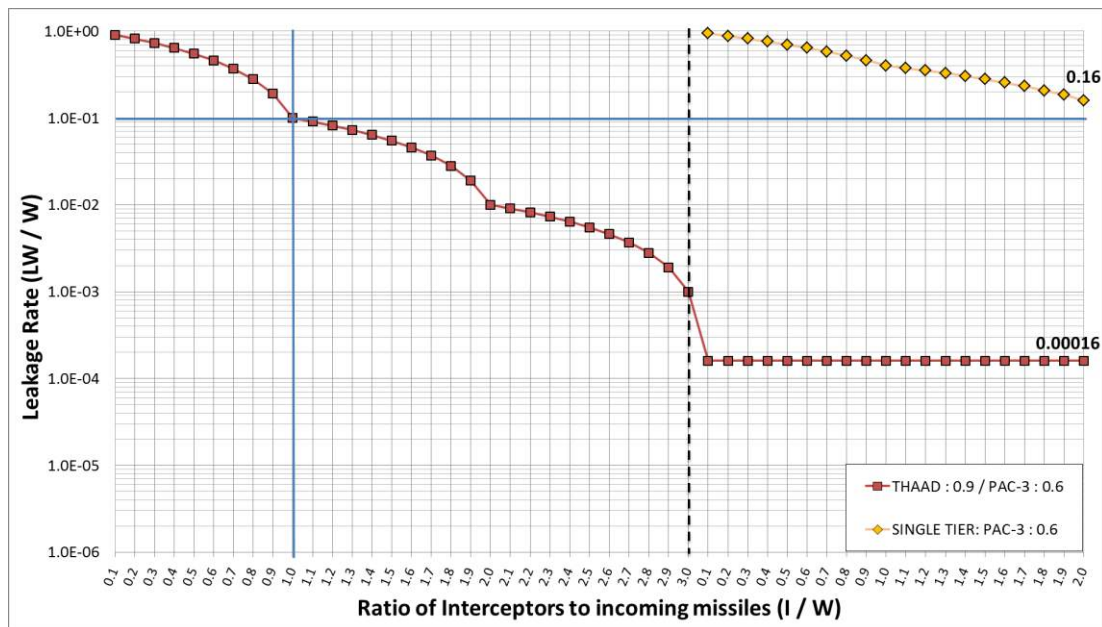
[그림 21] 사드: 3 발, PAC-3: 2 발 (SSPk: 0.9, 0.6, W=100)
