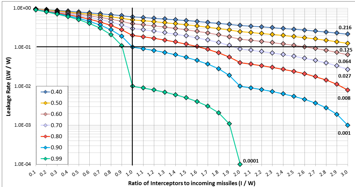
[그림 25] Tier-1 에서 SSPk 와 최대 3 발의 요격미사일 수에 따른 leakage rate 그래프
