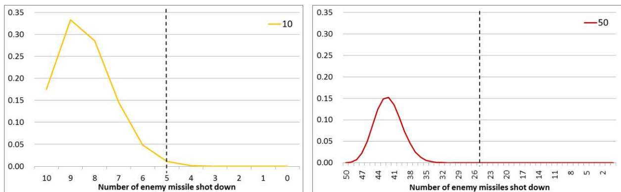
[그림 18] Tier-1 에서 격추된 적 미사일 수에 대한 확률분포 (W=10, 50)
