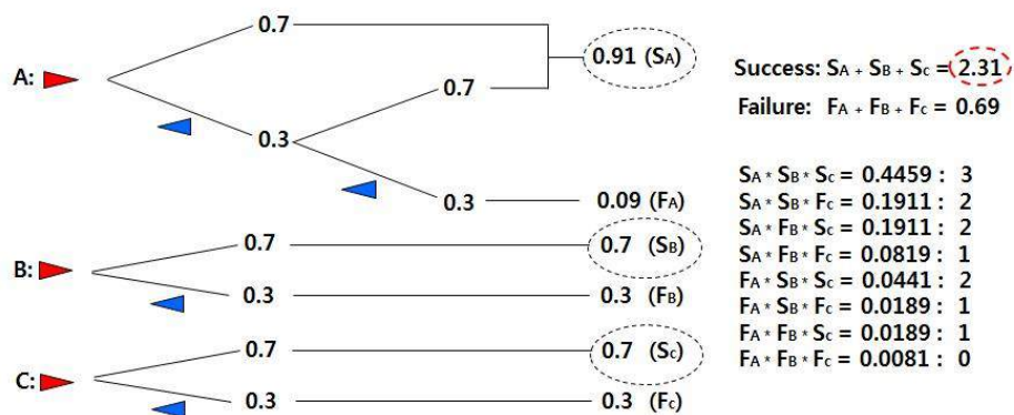
[그림 7] Tier-1 의 요격 성공과 실패 경우의 수와 확률
