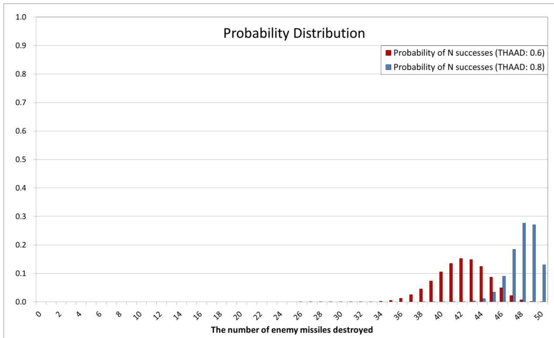
[그림 16] Tier-1 에서 격추된 적 미사일 수에 따른 확률분포
