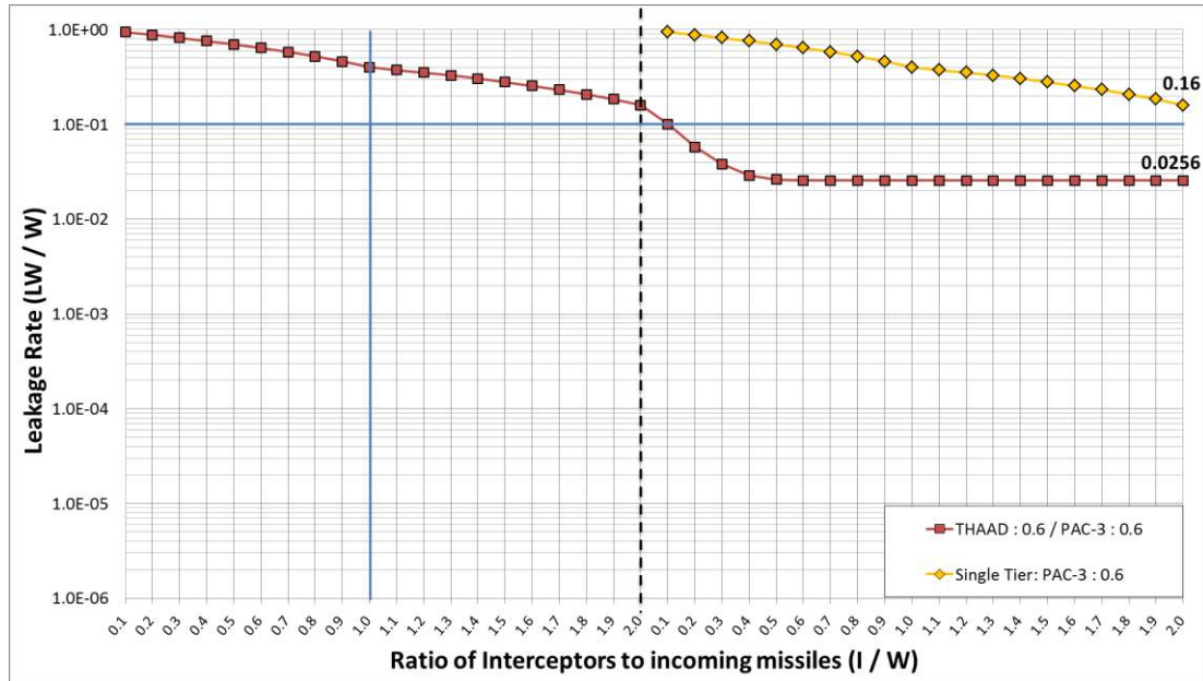
[그림 20] 사드: 2 발, PAC-3: 2 발 (SSPk: 0.6, 0.6, W=100) 46
