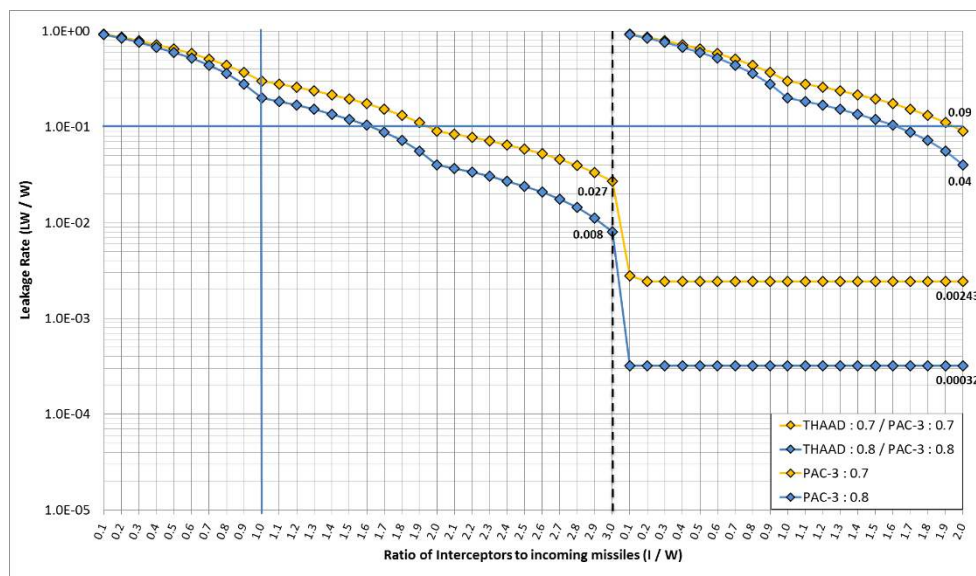
[그림 27] 사드: 3 발, PAC-3: 2 발 (SSPk: 0.7, 0.8, W=100)
