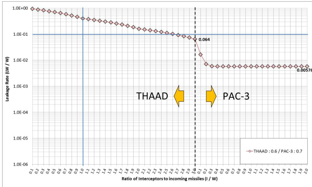
[그림 13] Tier-1 과 Tier2 의 leakage rate 그래프 (W=50)
