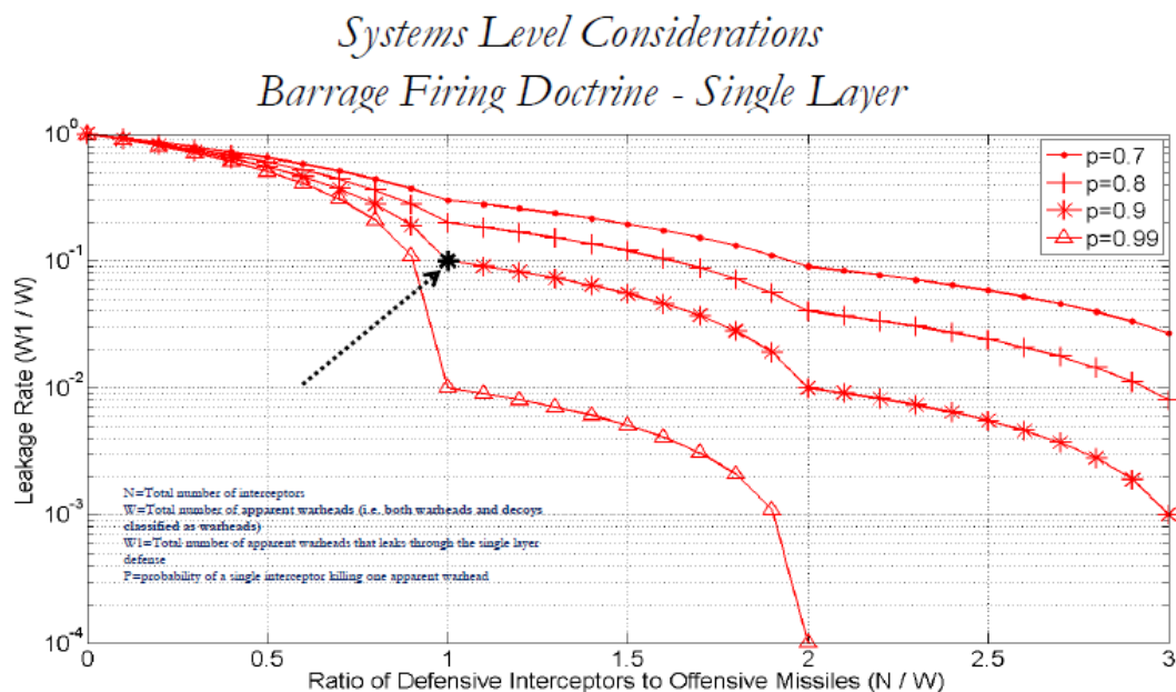
[그림 10] 단층 방어망에서 적 미사일 1 발 당 대응하는 요격미사일 수에 대한 leakage rate
