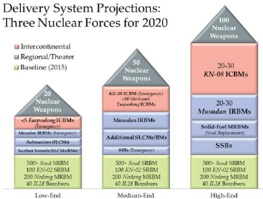
[그림 1] 2020 년 북한이 확보할 핵 미사일 규모에 대한 예측
