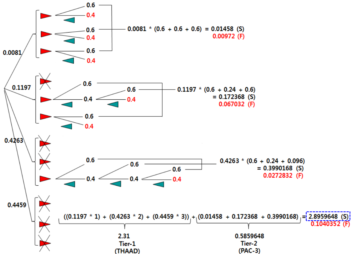
[그림 8] Tier-2 의 요격 성공과 실패 경우의 수와 확률
