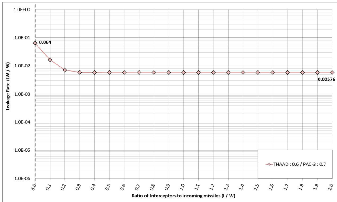
[그림 12] Tier-2 의 leakage rate 그래프 (W = 50)
