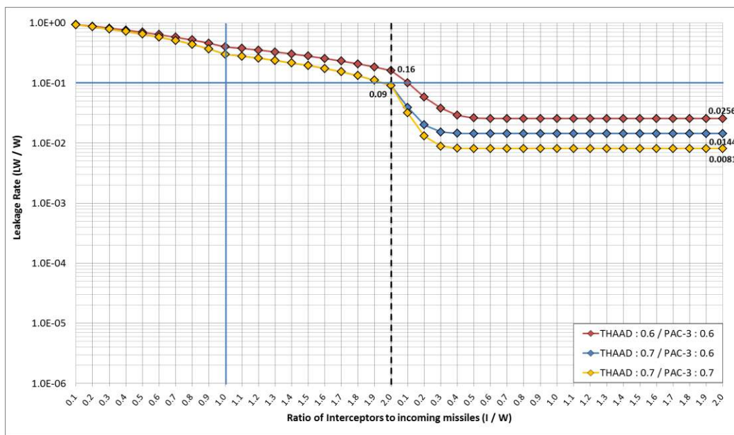
[그림 22] 사드: 2 발, PAC-3: 2 발 (SSPk: 0.6~0.7, W=100)
